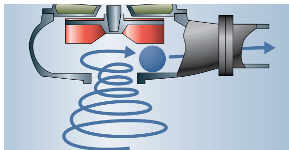
Hohe Zuverlässigkeit, geringe Abnutzung: Die leistungsstarke Pumpwirkung des Freistromrades ermöglicht den zuverlässigen Durchgang größerer Feststoffe
