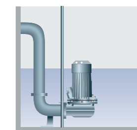
Stationäre Nassaufstellung: Mit schraubenlosem Kupplungssystem und Doppelführungsrohr
