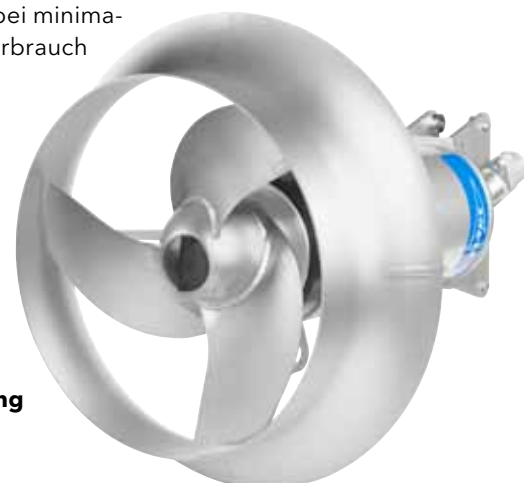
Optionaler Strömungsring.
